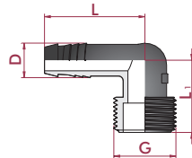
Gomito filetto maschio - portagomma
