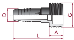
Manicotto filetto maschio - portagomma
